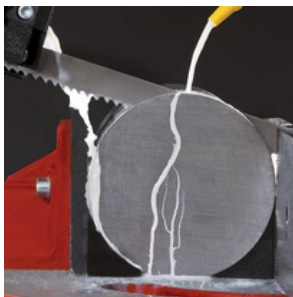
Bi-Metal
